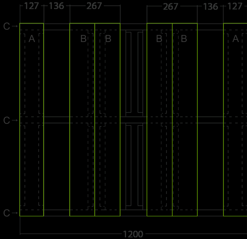
VISTA SUPERIOR
