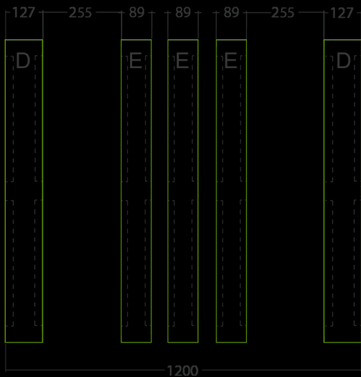
VISTA INFERIOR
